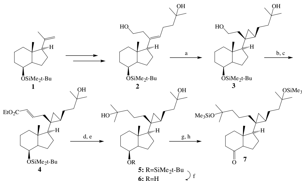
Scheme 1. Reagents: (a) Et 2 Zn, CH 2 I 2 , CH 2 Cl 2 ; (b) PCC, CH 2 Cl 2 ; (c) EtO 2 P(O)CH 2 COOEt, t -BuOK, toluene; (d) H 2 , Pd/C, AcOEt; (e) MeMgBr, Et 2 O; (f) H 2 SiF 6 , THF–CH 3 CN; (g) PDC, CH 2 Cl 2 ; (h) TMS-imidazole, CH 2 Cl 2 .
